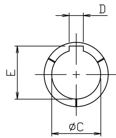
INPUT SHAFT
